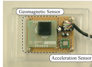
図 8 方位センサーユニット
