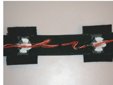
図 6 Active Belt ver.2 内部の配線 Fig. 6 Wiring inside of Active Belt ver.2
