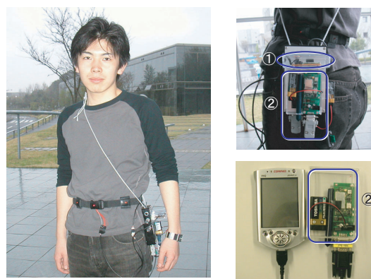
図 13 評価実験の様子。左:被験者, 右上:Active Belt 制御部, 右下:実験者操作部 (1. 方位センサー, 2. 無線シリアル送受信機)
