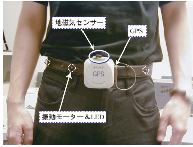
図 4 Active Belt ハードウェア ver.1 Fig. 4 Hardware of Active Belt ver.1
