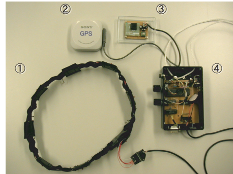
図2 Active Belt プロトタイプ (1. Active Belt ハードウェア, 2. GPS, 3. 方位センサーユニット, 4. 制御用マイコン) Fig. 2 Prototype system of Active Belt
