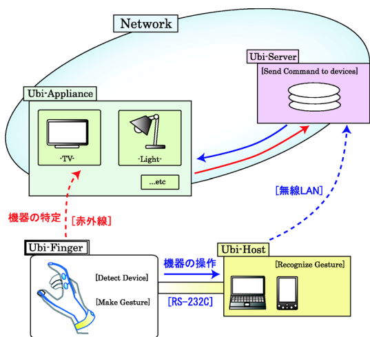
図 4 Ubi-Finger システム構成 Fig.4 System Configuration of Ubi-Finger
