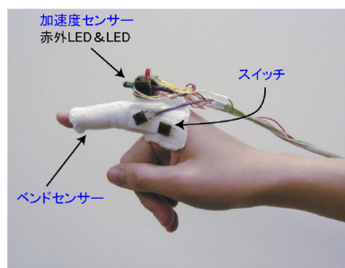
図 5 Ubi-Finger プロトタイプ Ver.2 Fig.5 Prototype of Ubi-Finger Ver.2
