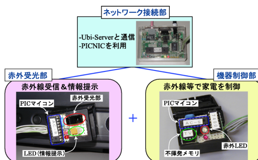
図 7 Attachable Controller システム図 Fig.7 System Configuration of Attachable Controller
