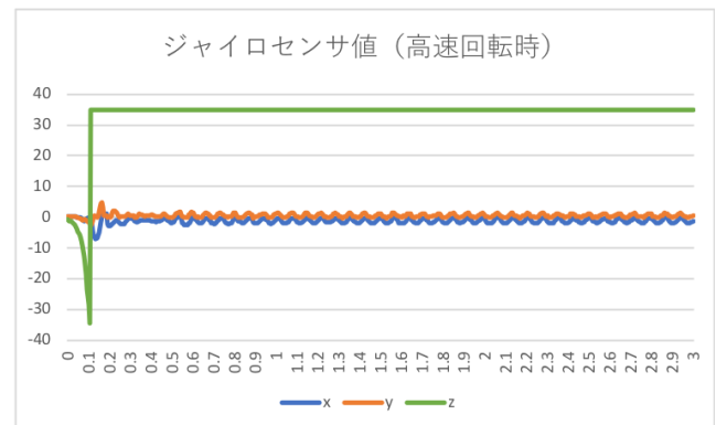
図 6 高速回転時のジャイロセンサ値
