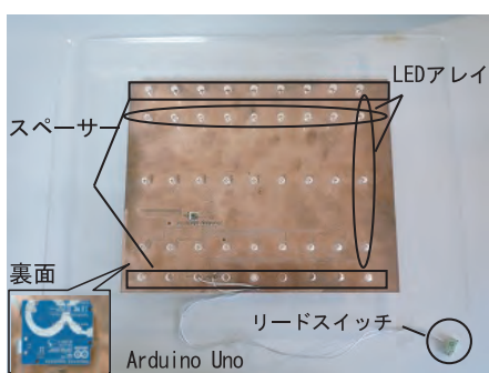
図 4 RefrigeMeter のデバイス構成 (左:プロトタイプ 1, 右:プロトタイプ 2) Fig. 4 Device Architectures of the RefrigeMeter(left:prototype1, right:prototype2)
